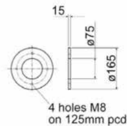
Site Flange
