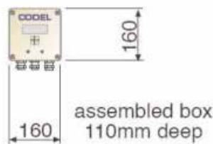
SPU/PSU (wt. 3kg)
